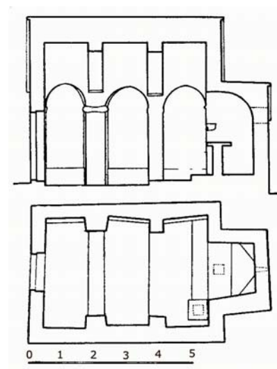
Presjek i tlocrt crkve Sv. Ilije
