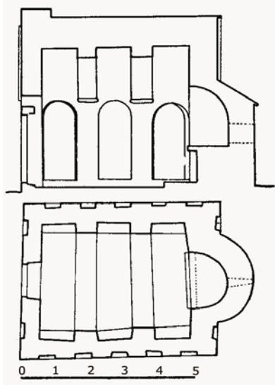
Presjek i tlocrt crkve Sv. Jurja
