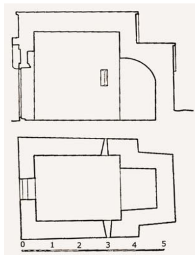
Presjek i tlocrt crkve Sv. Barbare
