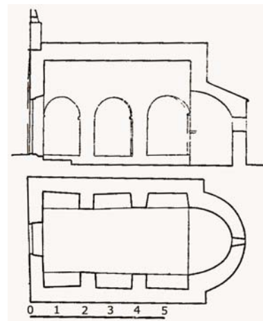
Presjek i tlocrt crkve Sv. Martina
