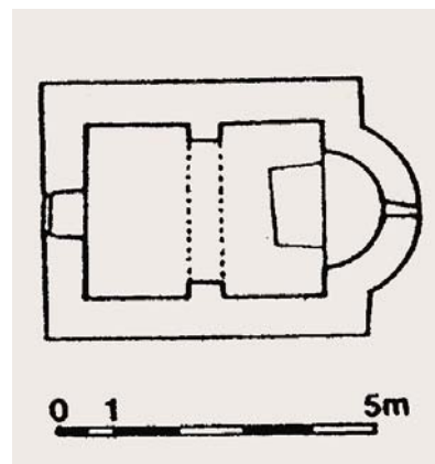
Tlocrt crkve Sv. Luke
