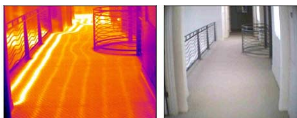
Slika 11. ICT provjera podnog grijanja
