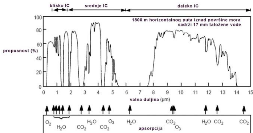
Slika 3. Atmosferski prozori [8]
