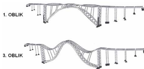
Slika 19. Prvi i treći proračunski modalni oblik titranja [7]
