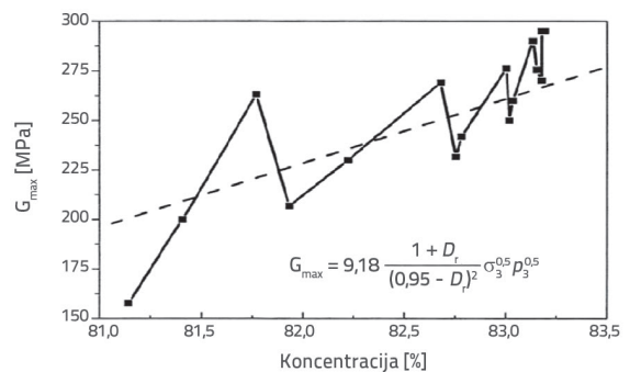
Slika 9. Odnos između modula posmika pri malim deformacijama i stupnjevima zbijenosti
