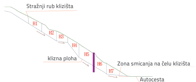
Slika 1. Zoniranje proračunskog presjeka klizišta
