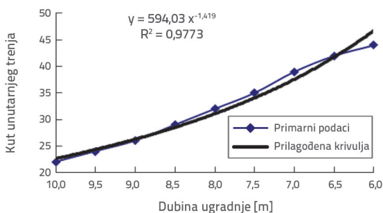
Slika 20. Krivulja odnosa između kuta unutarnjeg trenja φ i dubine ugradnje h u ukopnome dijelu tla
