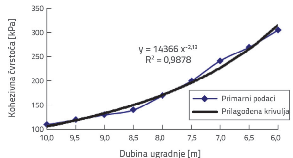
Slika 21. Odnos između kohezije tla c i dubine ugradnje h u ukopnome dijelu
