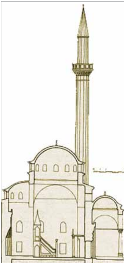
Poprečni presjek kroz građevinu
