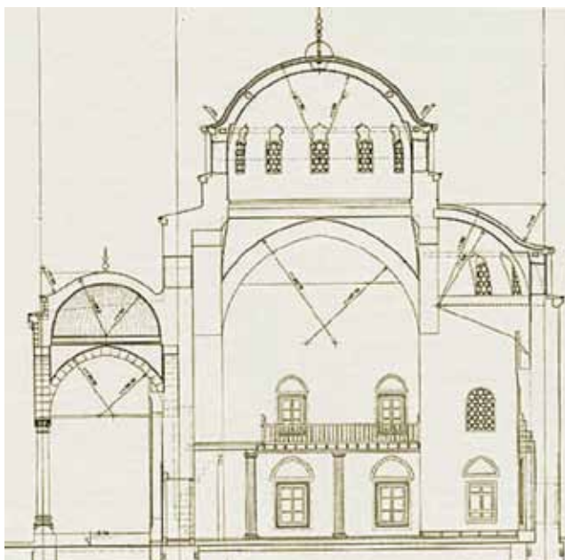
Uzdužni presjek kroz džamiju
