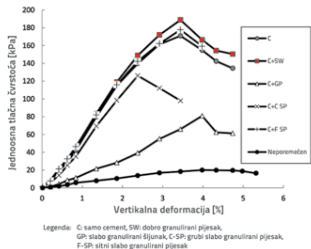
Slika 5. Odnos jednoosne tlačne čvrstoće i vertikalne deformacije uzoraka stabiliziranoga vlaknastog treseta
