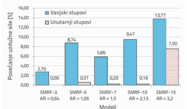
Slika 10. Povećanje uzdužne sile obodnih i unutarnjih stupova zbog primarnog udara
