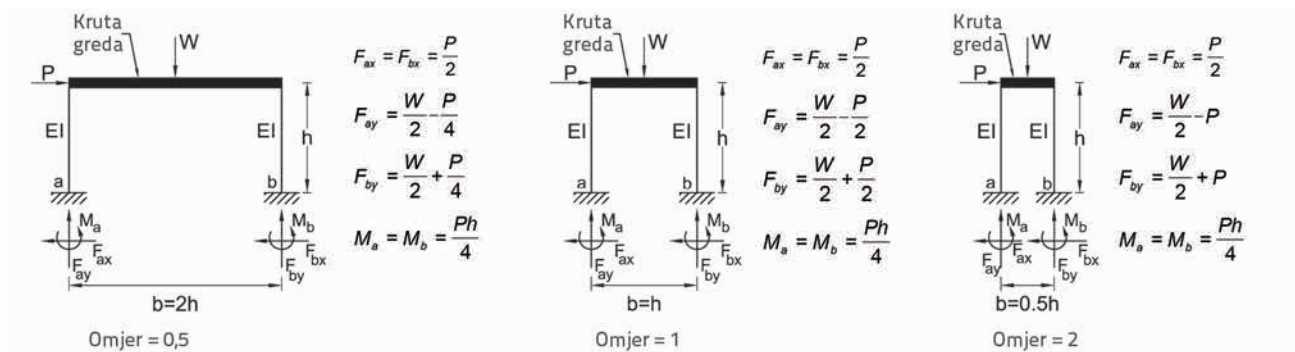
Slika 9. Usporedba promjene uzdužne sile stupova okvira i momenta savijanja sustava s jednim stupnjem slobode u odnosu na promjenu omjera visine i raspona
