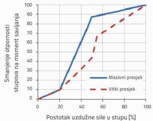
Slika 15. Promjena momenta savijanja u odnosu na uzdužnu silu
