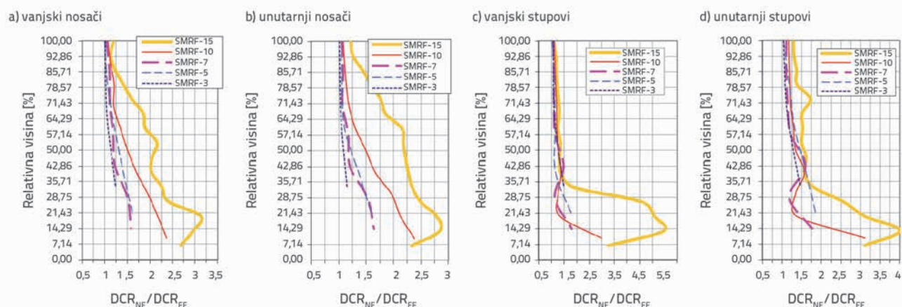
Slika 20. Odnos opterećenja i otpornosti (DCR) za bliski (NF) i udaljeni (FF) rasjed za elemente konstrukcije po visini modela
