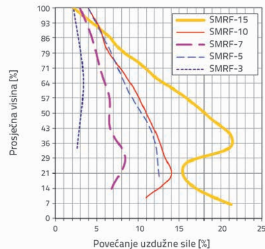
Slika 11. Povećanja uzdužnih sila obodnih stupova modeliranih katova
