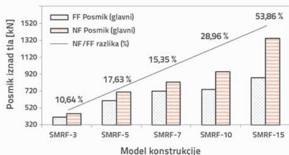
Slika 5. Usporedba prosječnih rezultata posmika iznad tla u bliskom i udaljenom području rasjeda
