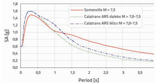
Slika 4. Usporedba spektara odziva ubrzanja rasjeda, \zeta = 5\% [24]
