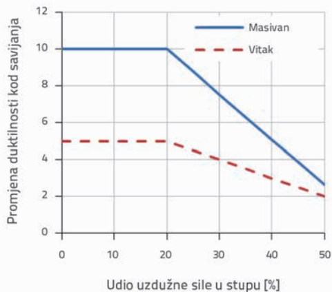
Slika 18. Promjena duktilnosti kod savijanja u odnosu na promjene uzdužne sile
