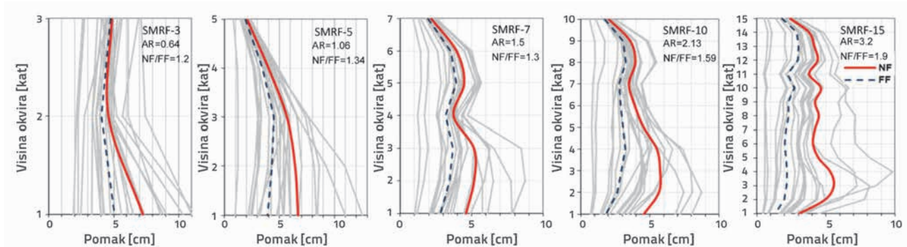
Slika 7. Usporedba srednjih rezultata zahtjeva za međukatnim pomakom u bliskim i udaljenim područjima rasjeda
