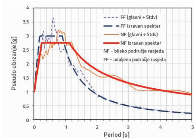
Slika 3. Izravnani spektri odziva rasjeda, \zeta = 5\%
