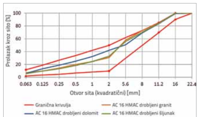
Slika 2. Granulometrijska krivulja agregata za izradu asfaltnih mješavina HMAC-a
